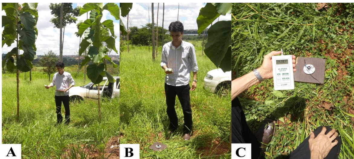
Figura 1. Determinação da incidência de radiação a 1,5 m do solo (A) e ao nível do solo (B) utilizando sensores de radiação fotossinteticamente ativa (C), Goiânia, GO, 2015.
